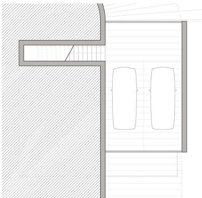
PLANTA SEMISOTERRANI
